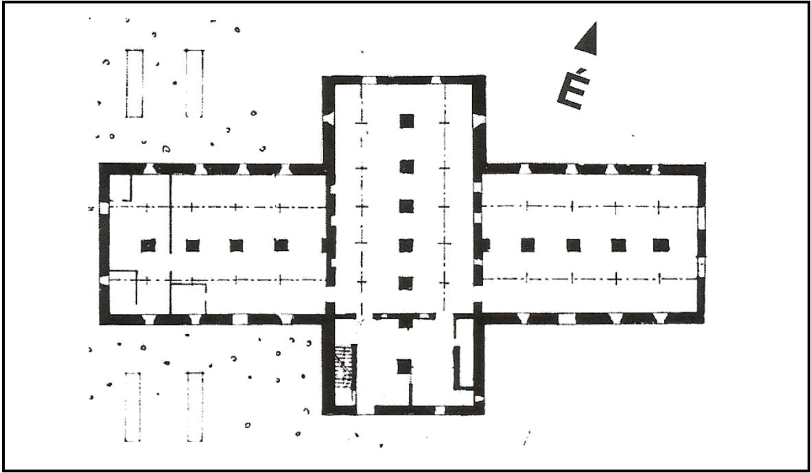
Alaprajz M 1:500
